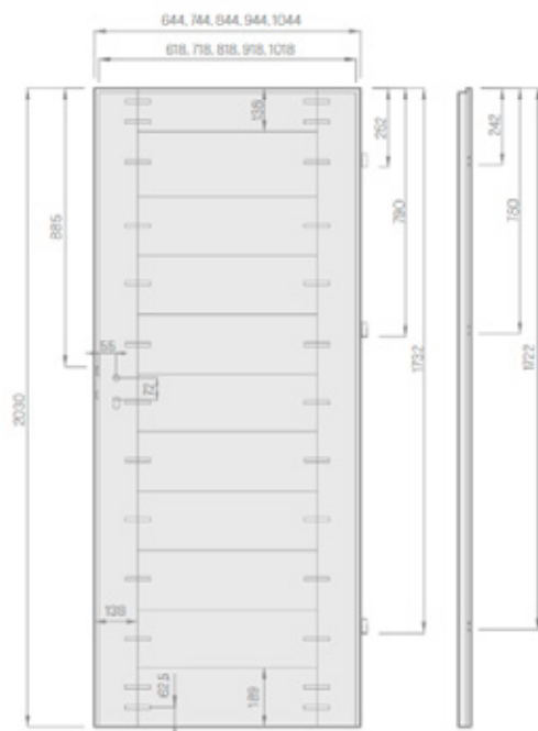
aanslag schuifraam
