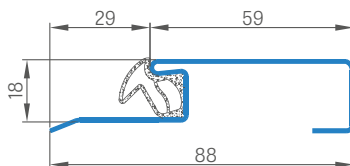
Roestvrij stalen drempel
