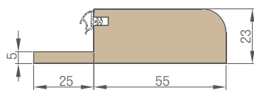
Hardhouten drempel
